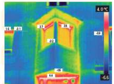
Zwei Beispiele von Thermographien: Visualisierung der Energieverluste
